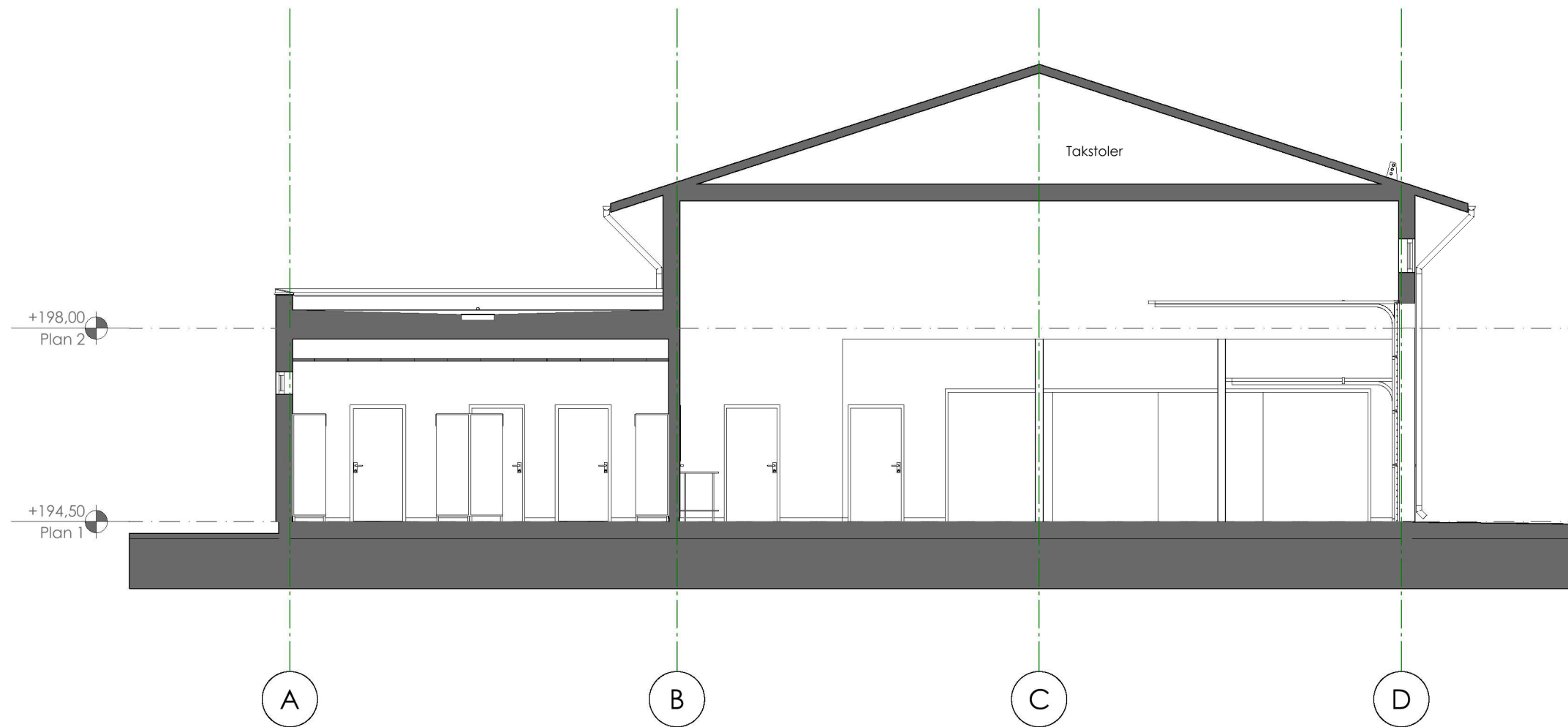
Snitt A
